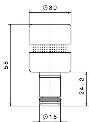
Giunto Filtrante Con 1 Filtro
